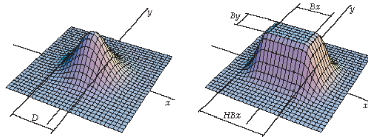
Bild 7. Typische Laserstrahlungsprofile
